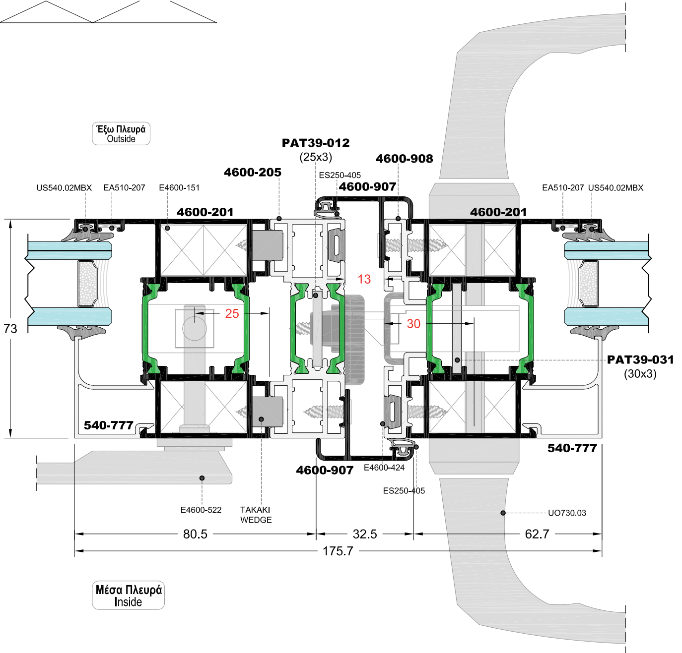
ΚΑΤΩΨΗ TOP VIEW
